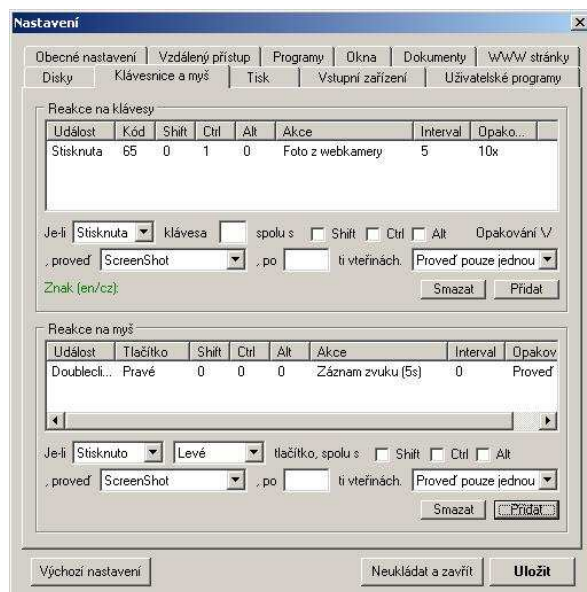
Nastavení klávesnice a myši
