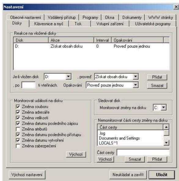
Nastavení sledování souborového systému
