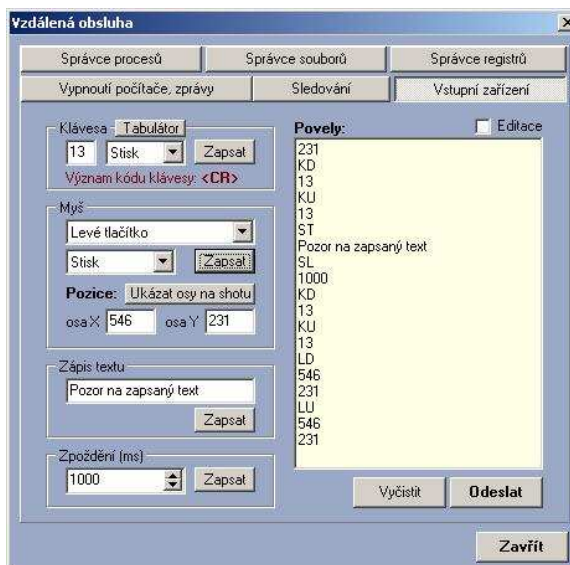
Zaslání stisků kláves, textu a kliků myši
