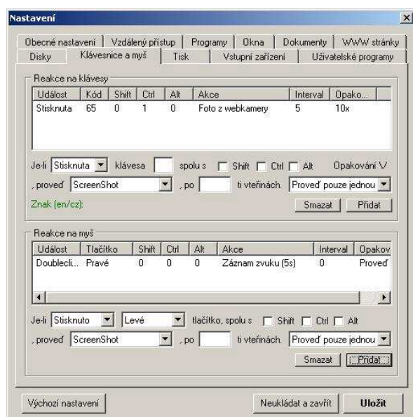
Nastavenie klávesnice a myši
