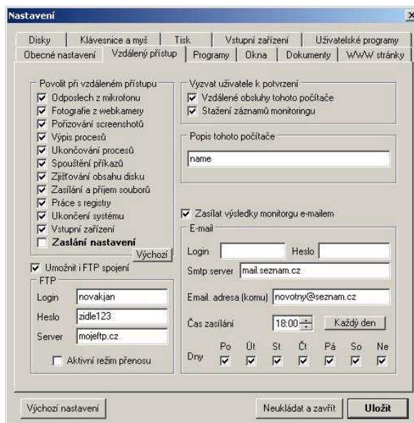
Nastavenie vzdialeného prístupu
